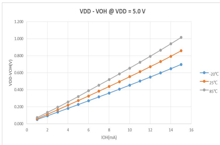
Figure 3-1 ( V_{DD} - V_{OH} ) 温度曲线
