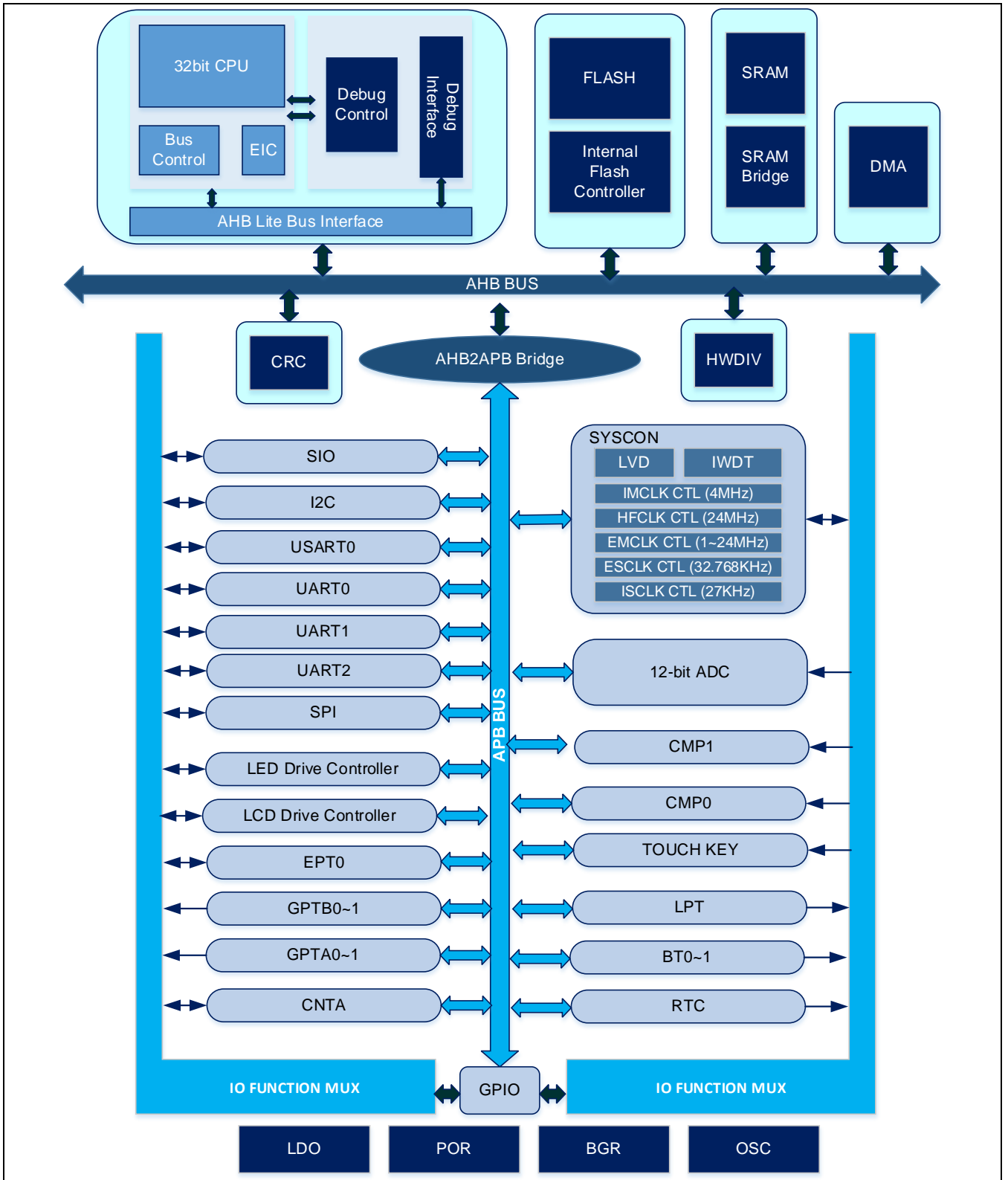
Figure 1-1 APT32S7108模块框图
