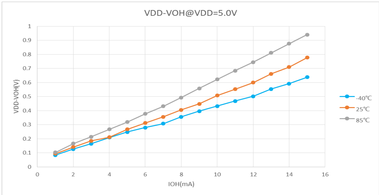
Figure 3-1 (VDD-VOH) 温度曲线
