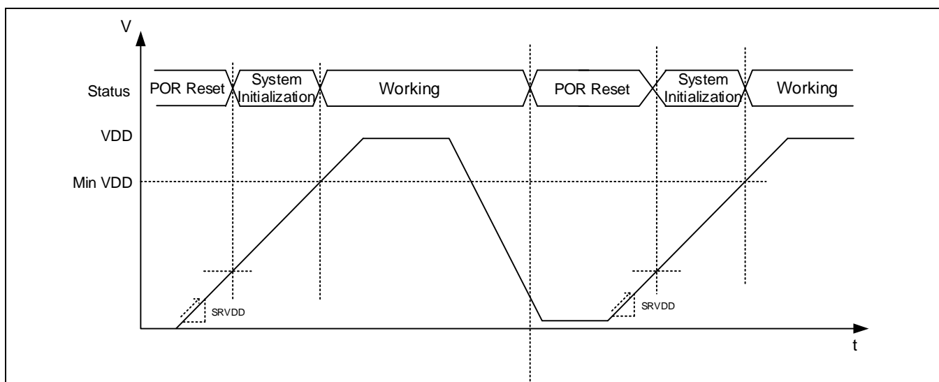
Figure 3-5 上电和掉电示意图
